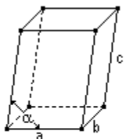
MONOCLINIC
